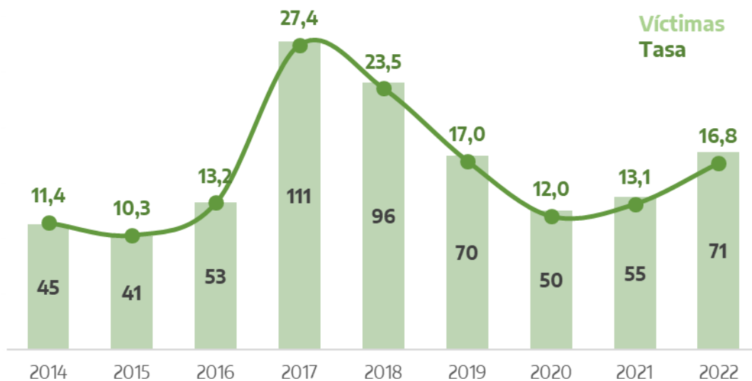
Gráfico 16. Víctimas de muertes en accidentes viales por año. Valores absolutos y tasas cada 100.000 habitantes. Provincia de Catamarca. Años 2014-2022
